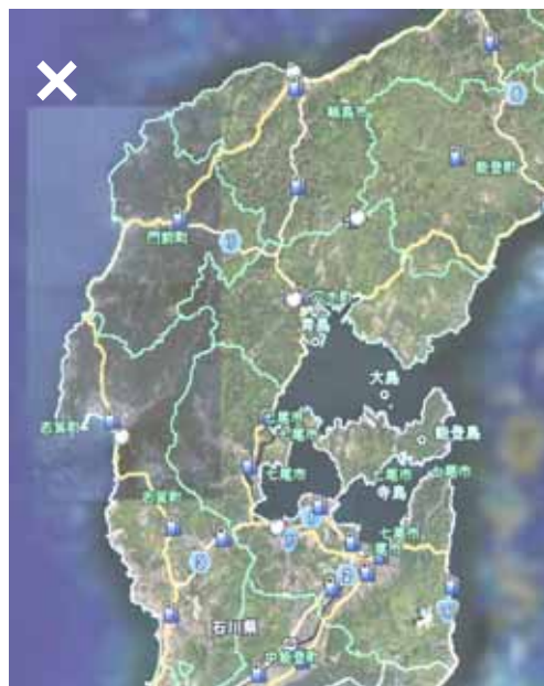
石川県能登半島地震震源地
